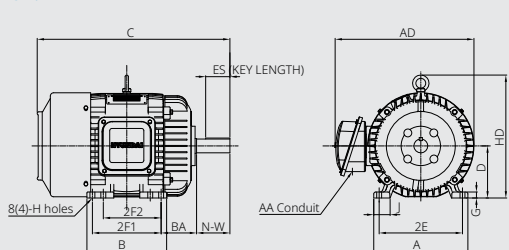
Fig. C 254 - 326Fr.
