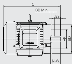
Fig. C 254 - 326Fr.
