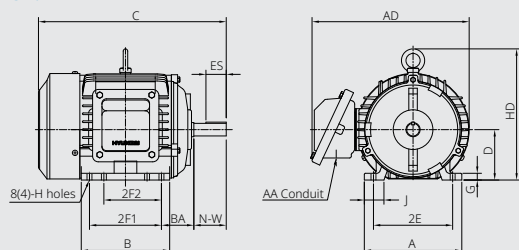
Fig. C 254 - 326Fr.
